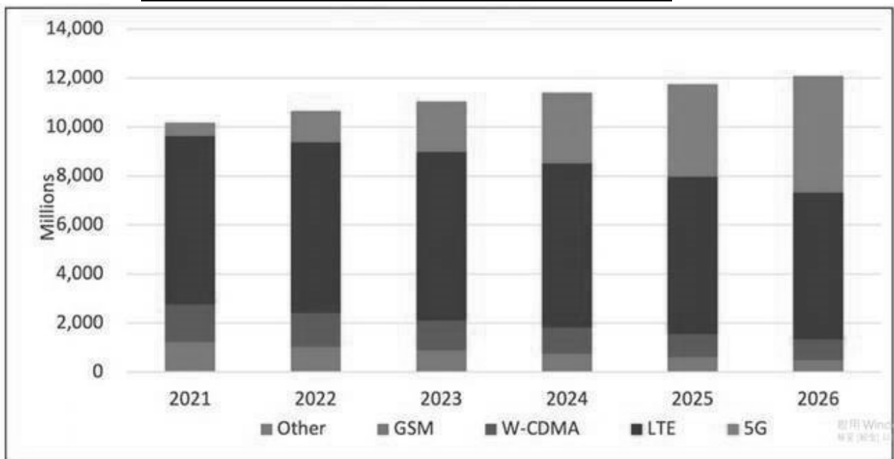
預估 2021~2026 年期間不同行動通訊技術用戶數之變化
